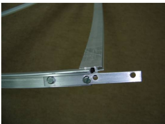
Fixação das longirinas nos beirais
