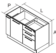
GB 1P4G-120 ST PRODUTO MONTADO: A: 830 L: 1199 P: 585 MM
