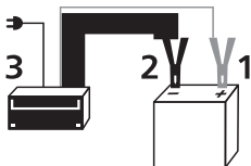
Figura 2 -Secuencia para encender el cargador en la batería
