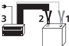
Figura 2 -Sequência para ligar o carregador na bateria
