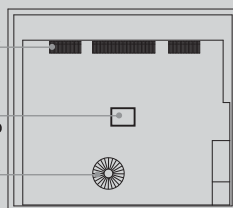
Vista do fundo do fogão cooktop por indução
