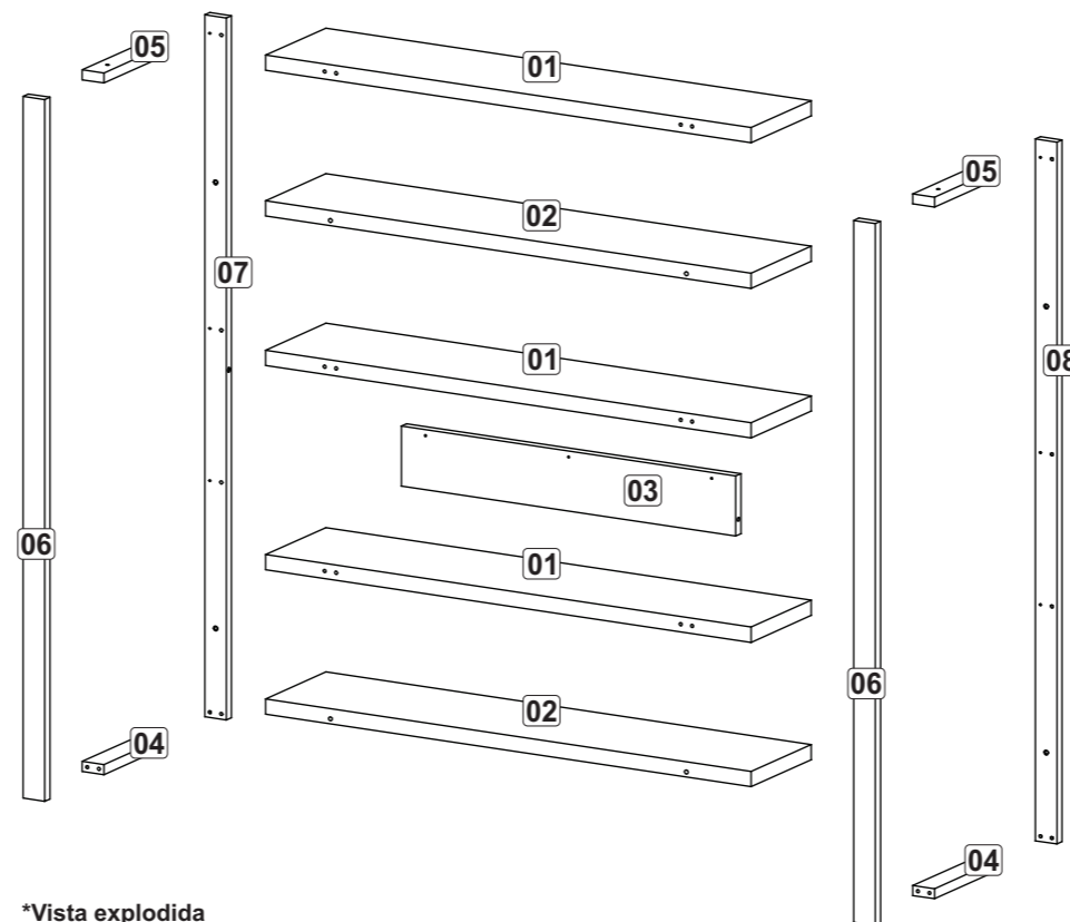
*Vista explodida
