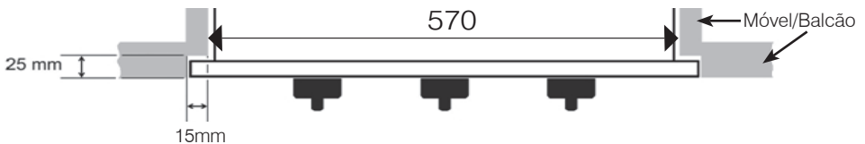
Figura 3.1 (forno todo embutido)
