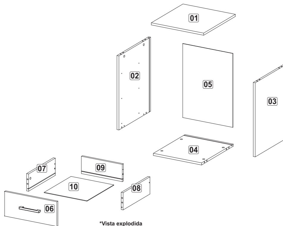
*Vista explodida
