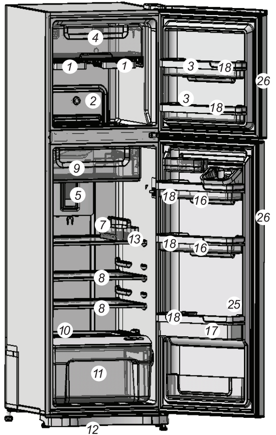
Modelo DF42/DF42X
