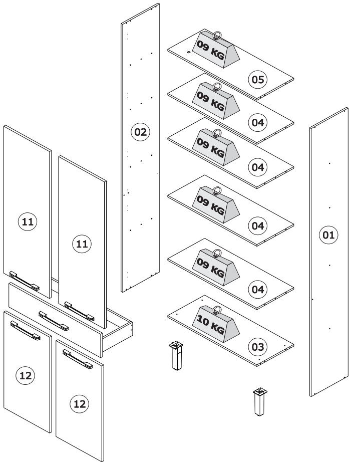
PAN-70 4PT1GAV PRODUTO MONTADO: A: 2000 L: 700 P: 300 MM
