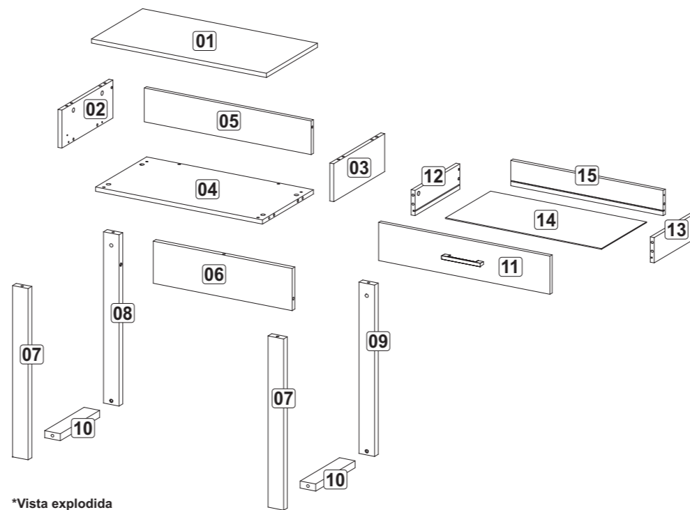
*Vista explodida
