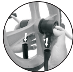
1.3 - Encaixe os mancais no tubo do garfo.
