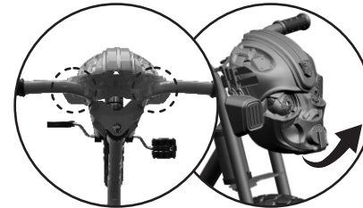
3.2 - Posicione a máscara à frente do guidão do produto e encaixe as travas, conforme ilustração. Para remover, puxe a máscara por baixo (item de acordo com o modelo adquirido).
